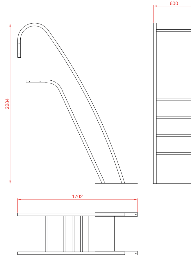
Dimensiones generales (en milímetros)
